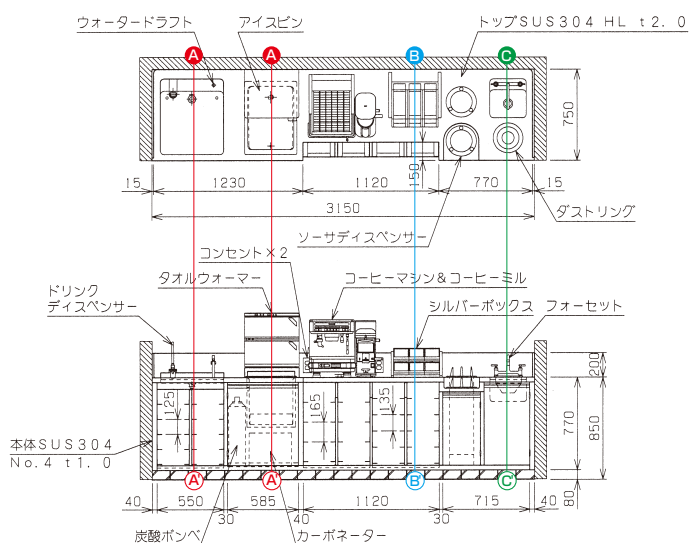
正面図／上面図
