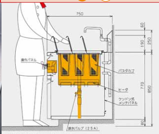
配置 D—D
