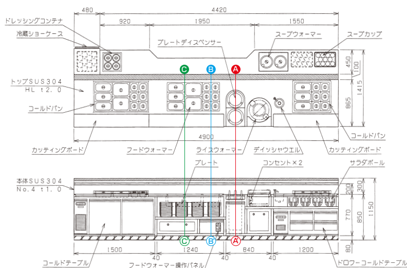
正面図／上面図
