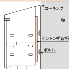
取付方法
