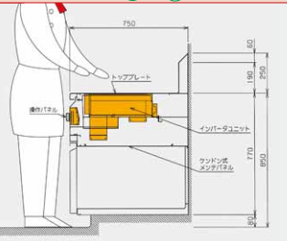
配置 C—C
