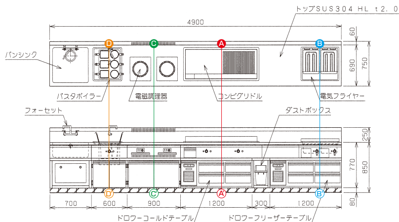
正面図／上面図
