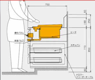
配置 B—B
