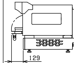
オ - プン扉開時寸法
